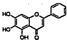
BAICALEIN
